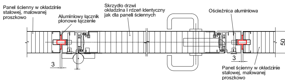
C-C
